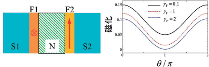
図. 2 超伝導体(S), 強磁性体(F)そして常磁性体(N)から構成される多重接合(左の図)で, スピン三重項クーパー対のスピンによってNに誘起される磁化のS間の位相差の依存性(右の図)
