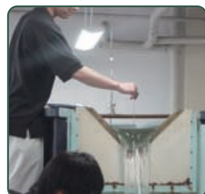
水理実験 Hydraulics Experiment
