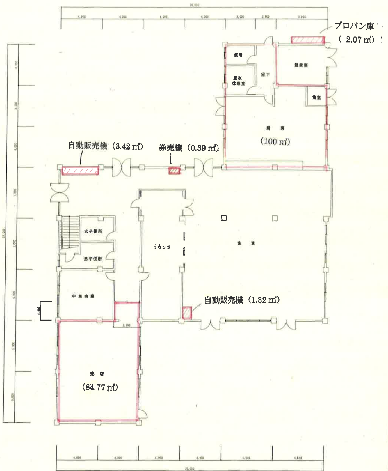
福利施設 1階平面図 S=1:100
