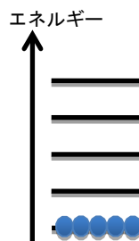
図1：ボソン
