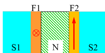
図.2 超伝導体(S)、強磁性体(F)そして常磁性体(N)から構成される多重接合(左の図)で、スピン三重項クーパー対のスピンによってNに誘起される磁化のS間の位相差の依存性(右の図)
