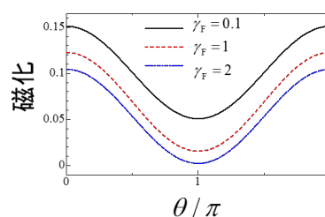
図.2 超伝導体(S)、強磁性体(F)そして常磁性体(N)から構成される多重接合(左の図)で、スピン三重項クーパー対のスピンによってNに誘起される磁化のS間の位相差の依存性(右の図)
