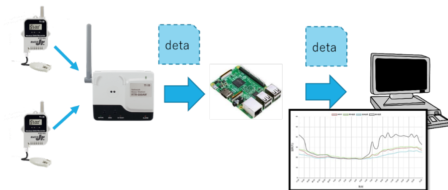
図1 マイコン等を用いたデータ計測
