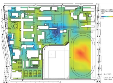
図2 温度情報の可視化
