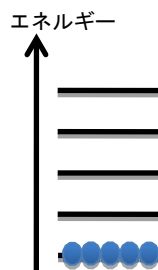
図1：ボソン
