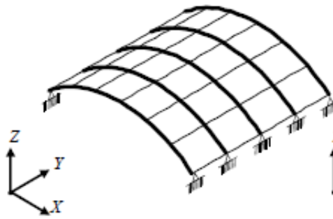
図2 円筒ラチスシェル
