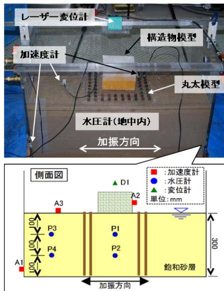
図1 対策工法の実験概要
