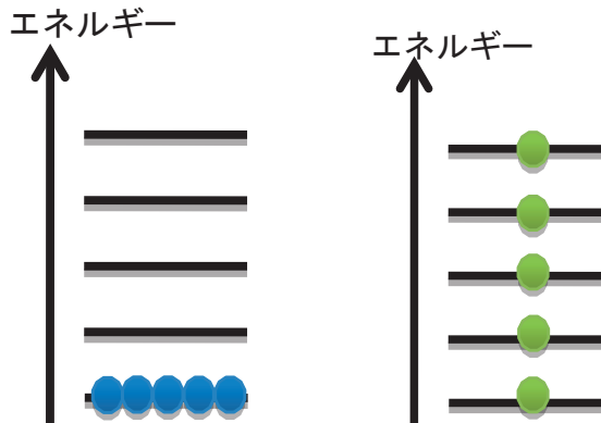
図1: ボソン
