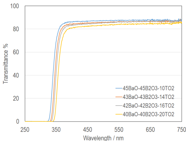
図 2 BaO-B 2 O 3 -TiO 2 ガラスの透過率スペクトル.
