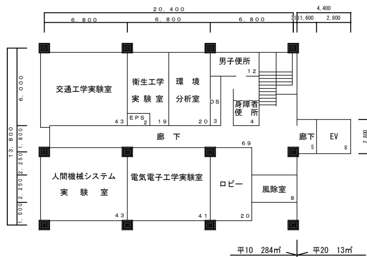
1 階
