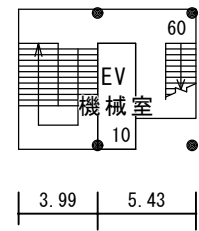
塔屋 1 階
