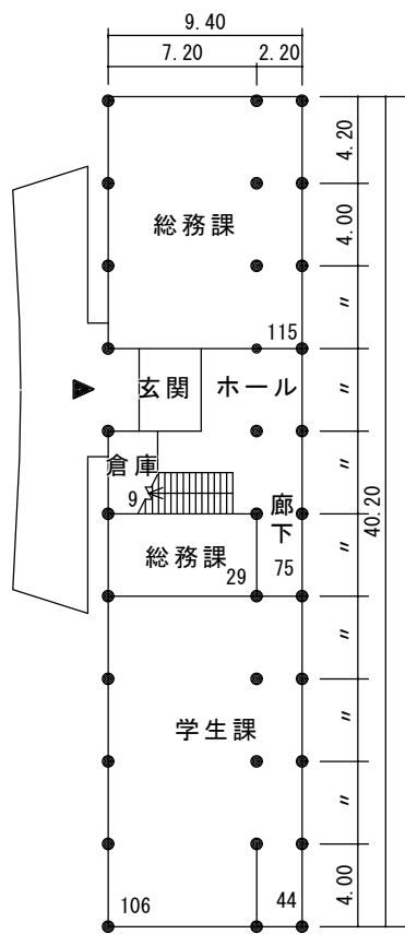
1 階
