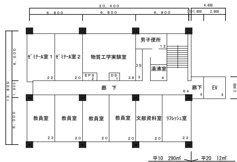
2 階
