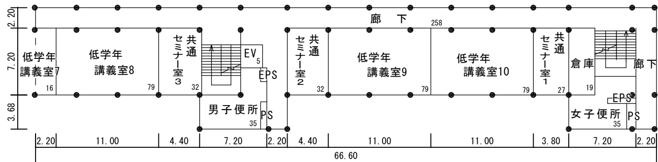
3 階
