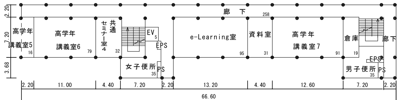
4 階
