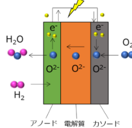
燃料電池の発電原理
