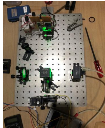
図 3. レーザー干渉計
