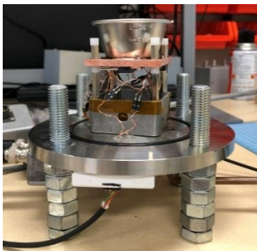
図 4. 熱放射測定系
