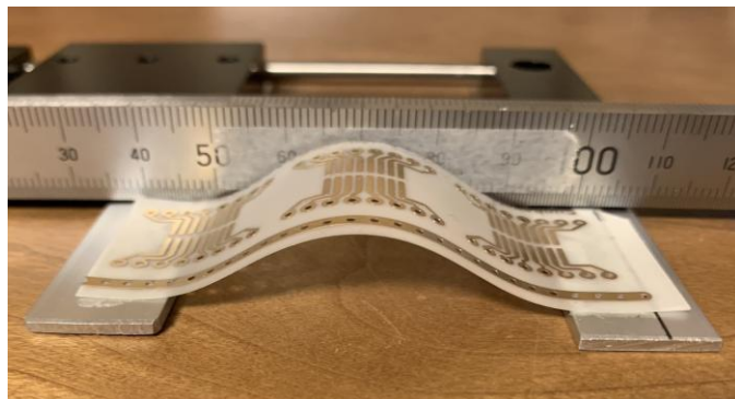
図 5. 歪印加装置
