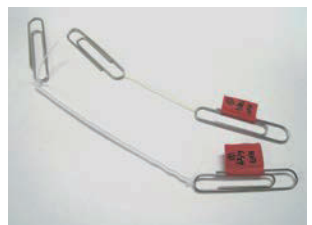
試作した人工筋肉 (右図)
